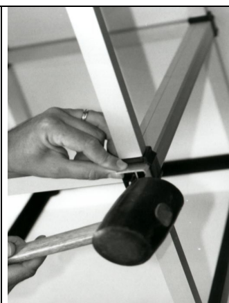
Montage de KIT-CAD 1.2 (Couplage)
