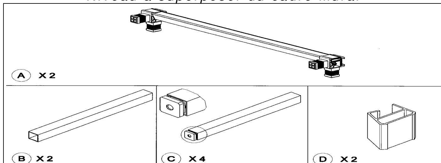
Cadre de classement modulable en hauteur
