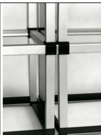
Montage de KIT-CAD 1.2 (Couplage)
