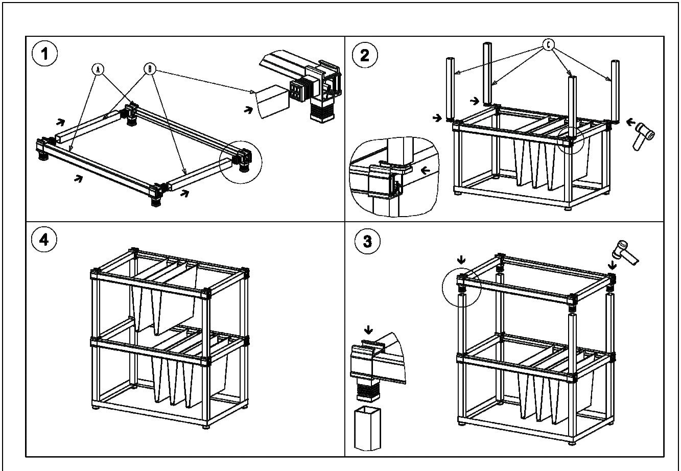
Montage du niveau KIT-CAD 1.2
