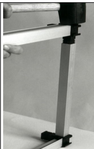
Montage de KIT-CAD 1.1
